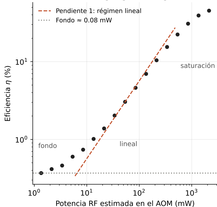
(b) Escala log-log: tres regímenes
