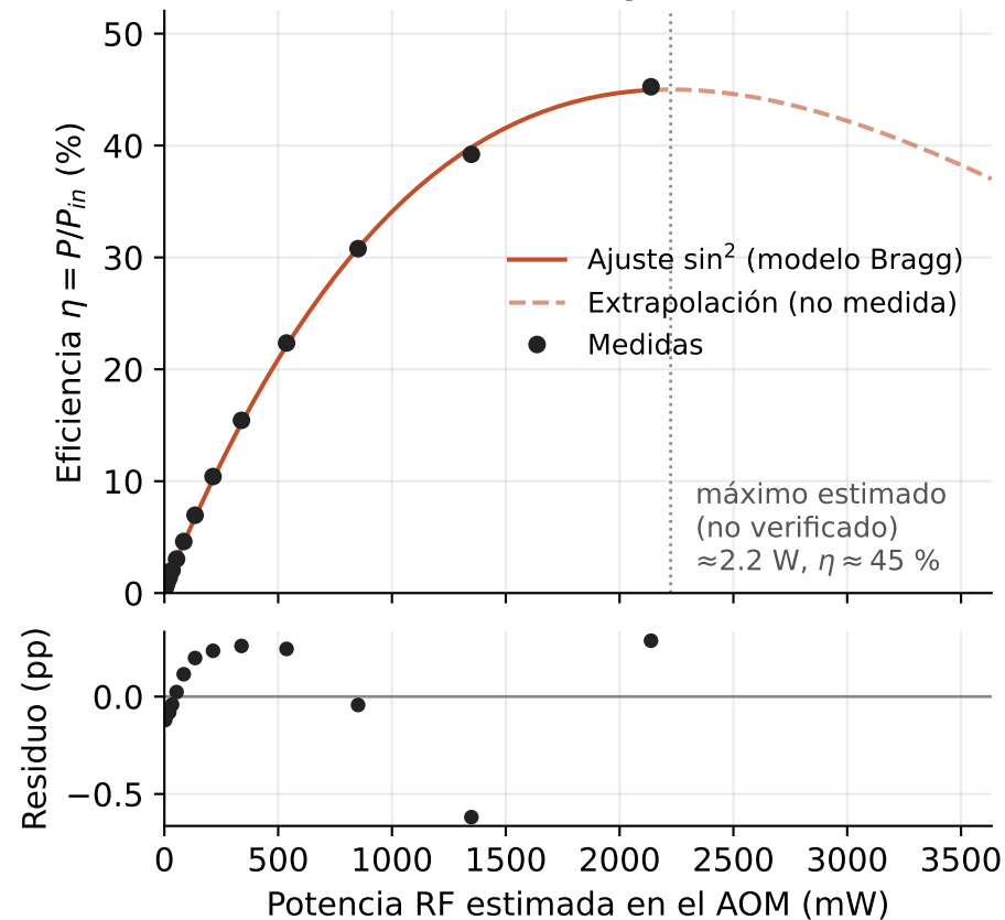
(a) Eficiencia vs potencia RF
